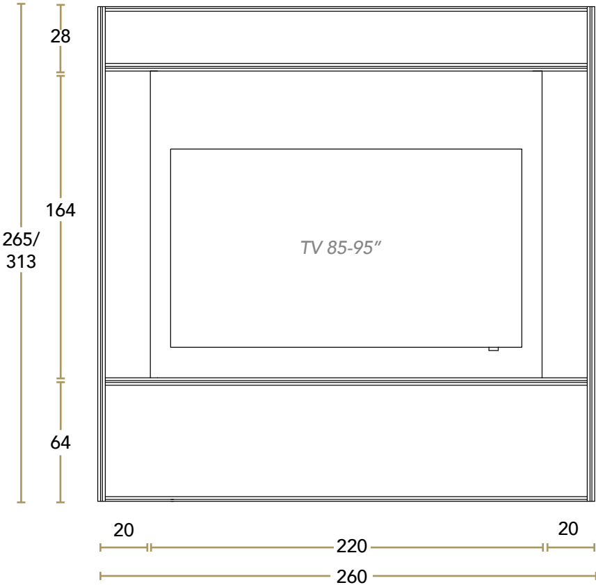
Modulo per TV da 85 - 95" 85 - 95" TV Module
