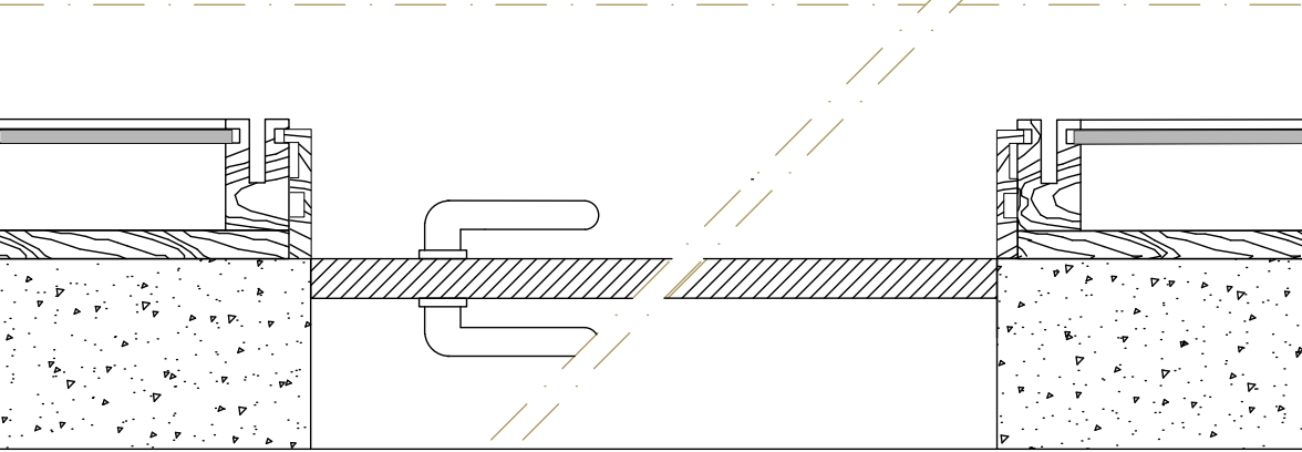
Sezione di un modulo passaggio Section of a pass - through module
