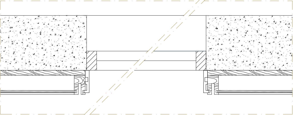
Sezione di un modulo finestra Section of a window module
