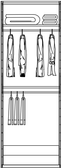
Coperchio Top element 2 Ripiani regolabili con tubo appendiabiti 2 Adjustble shelves with clothes rod Cassettiera fissa 2 cassetti 2 Fixed rrawer-unit Basameto Base basement
