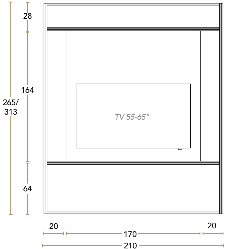
Modulo per TV da 55 - 65" 55 - 65" TV Module
