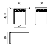
4009 Tavolino lato Side table
