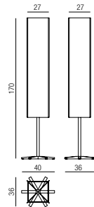
4007 Lampada da terra Floor lamp
