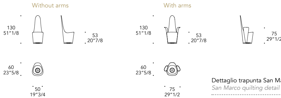
Interno trapuntato San Marco. Dotata di ruote. San Marco internal quilting. Equipped with wheels.
